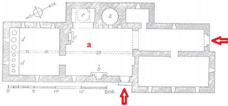
Şekil 17 Muradiye İmâreti planı (A. Gabriel)
