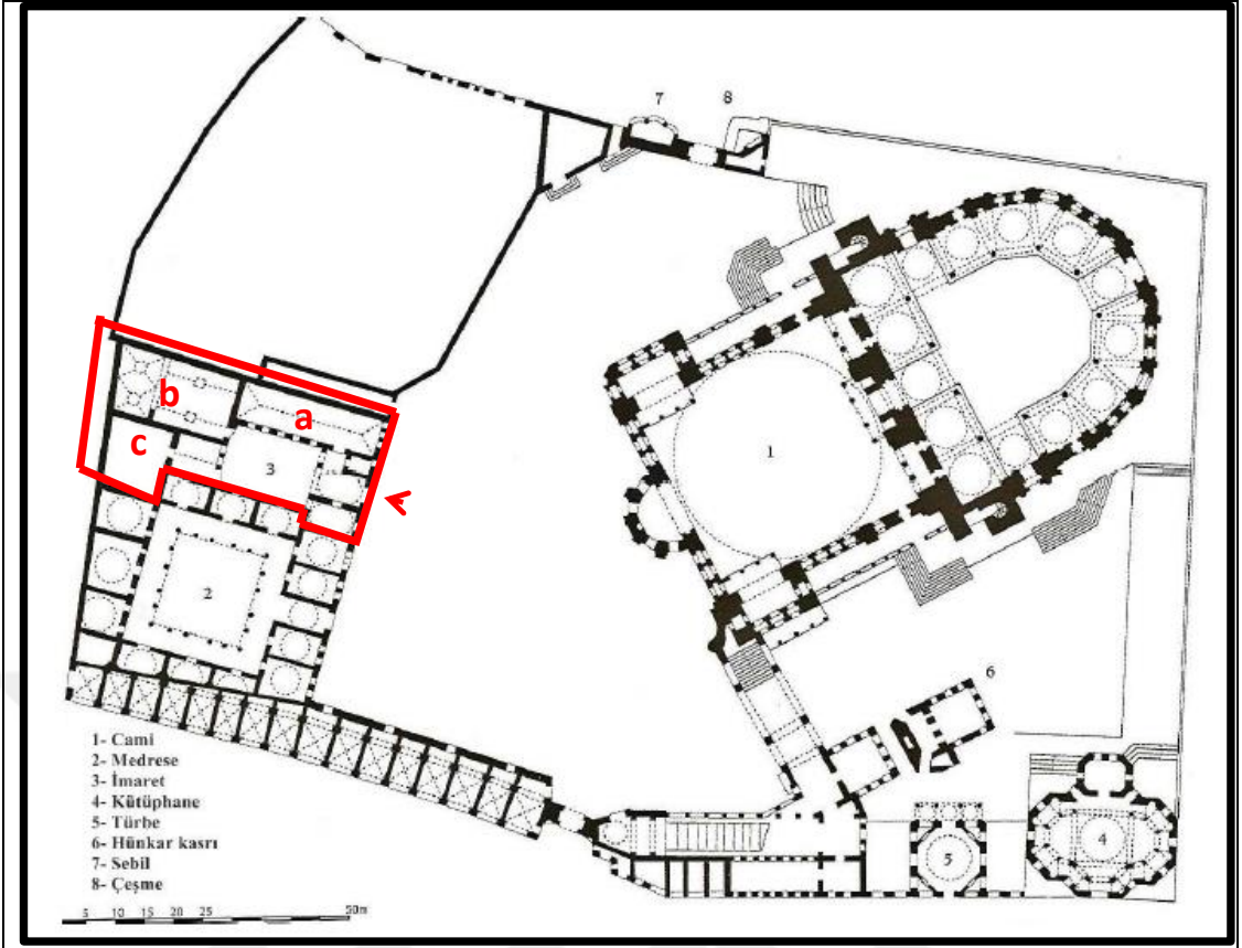
Şekil 136 Nuruosmaniye Külliyesi Vaziyet Planı (Doğan KUBAN)
