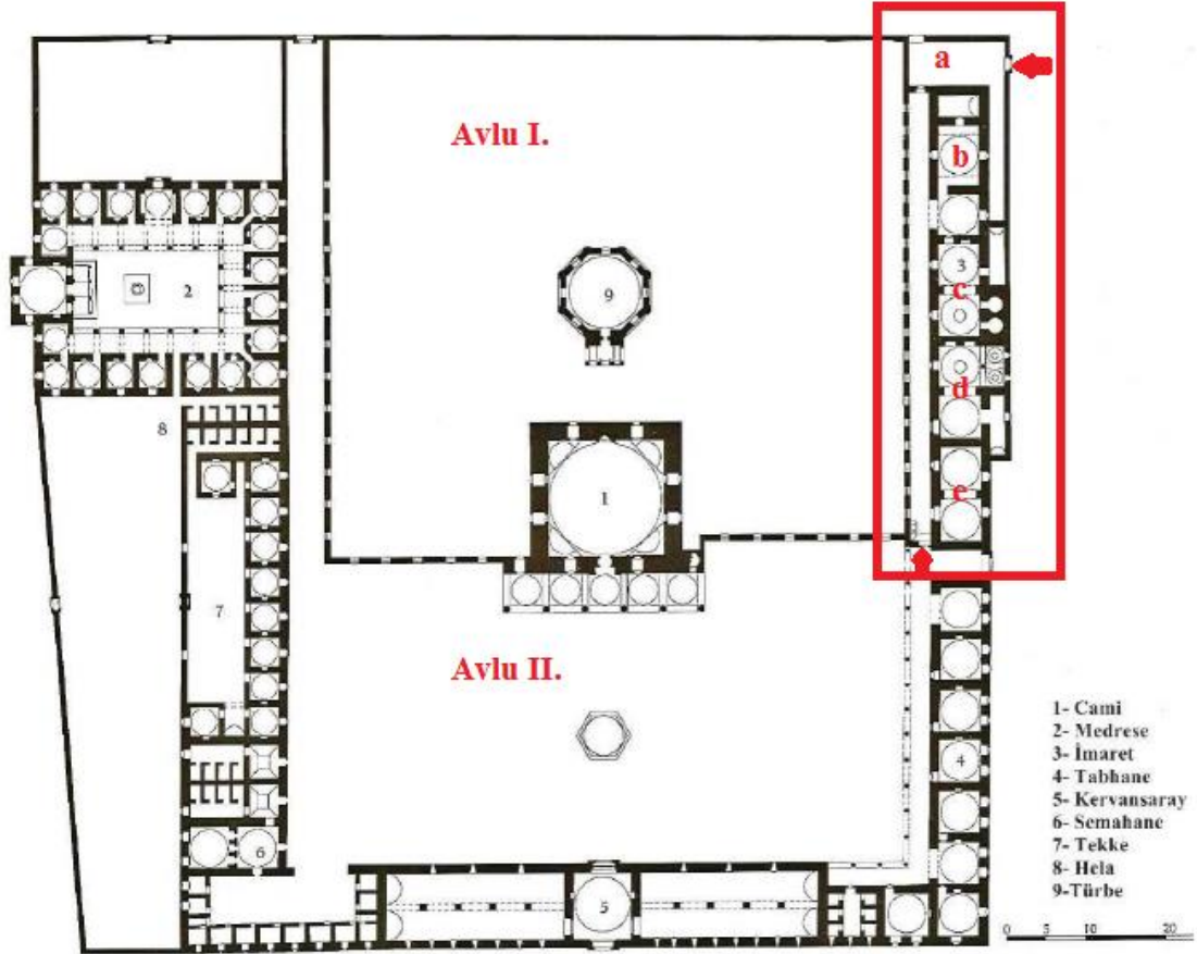
Şekil 41 Gebze Çoban Mustafa Külliyesi Vaziyet Planı (A. Kuran)
