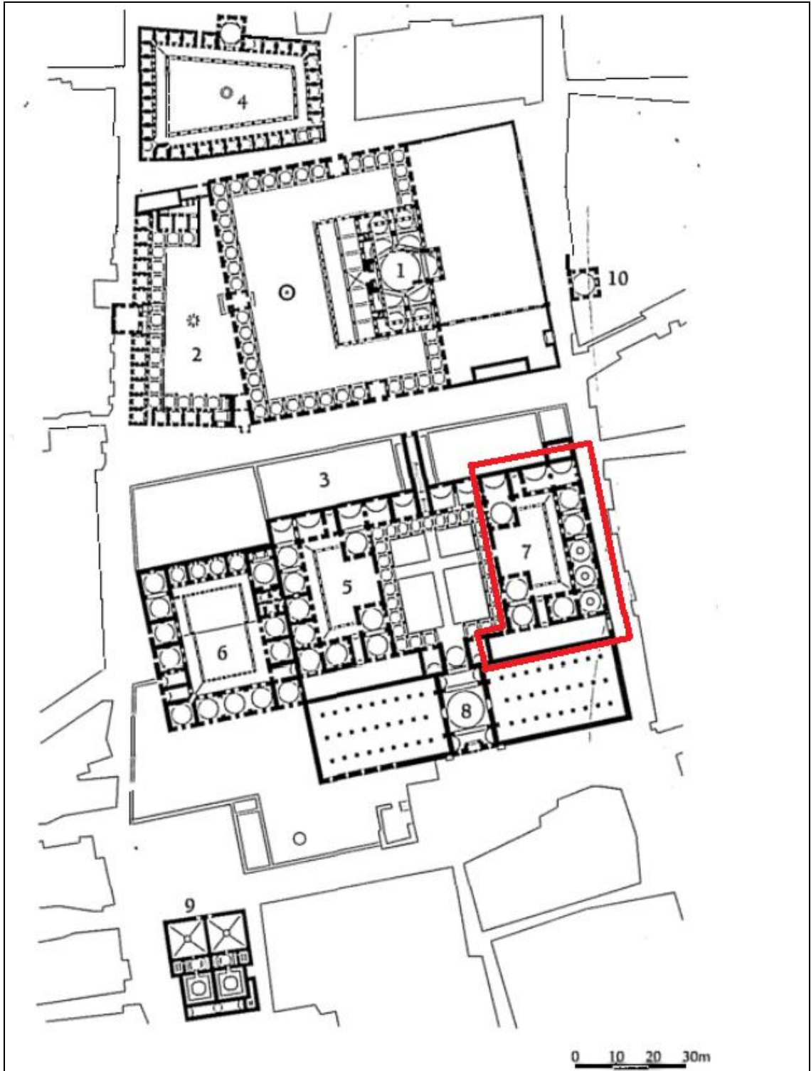
Atik Valide Külliyesi, Üsküdar, İstanbul. Yerleşim planı: 1. Cami, 2. Medrese, 3. Dârülhadis, 4. Tekke, 5. Tabhane, 6. Dârüşşifa, 7. İmaret, 8. Kervansaray, 9. Hamam, 10. Sibyan Mektebi (A. S. Ülgen)
