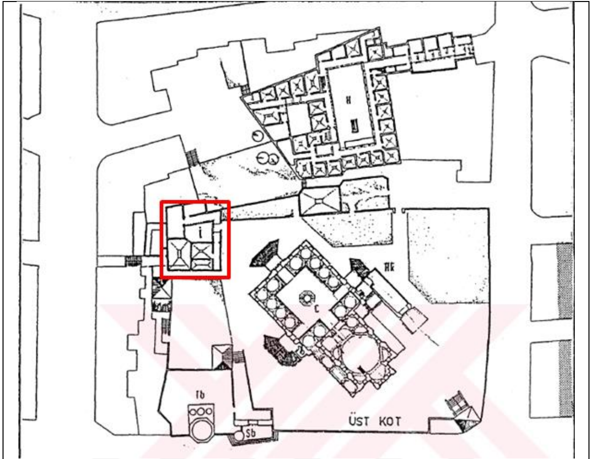
Şekil 144 Laleli Külliyesi Vaziyet Planı (Aras Neftçi)
