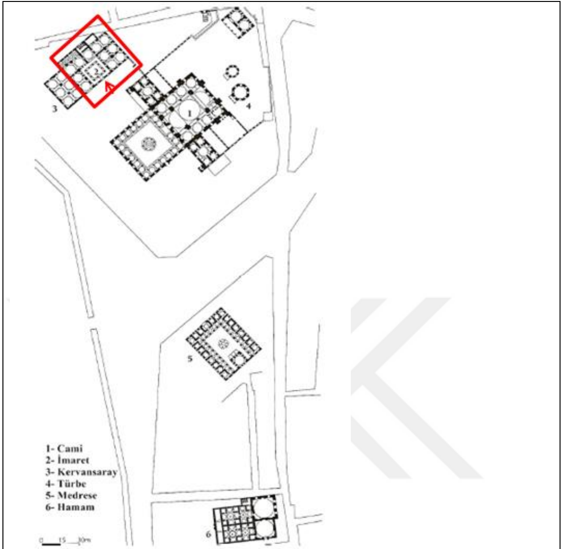
Şekil 31 II. Bayezid Külliyesi (İstanbul) Vaziyet Planı (A. Yüksel)
