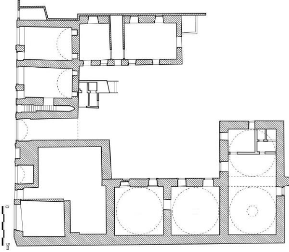
Şekil 109 Gölmarmara Halime Hatun İmaret (Ş. Çakmak'tan)
