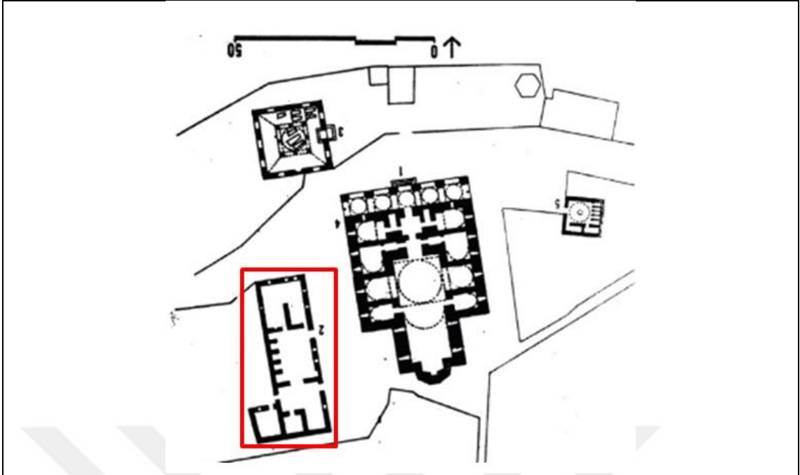
Şekil 159 Hüdavendigâr Külliyesi Vaziyet Planı ( http://www.sehrinesesver.com/sehir/toplumu-ve-dogayi-ilmek-ilmek-dokumus-bir-kent-bursa/ )
