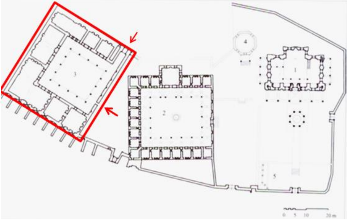
Şekil 104 Manisa Muradiye Külliyesi Vaziyet Planı (Gülru Necipoğlu)
