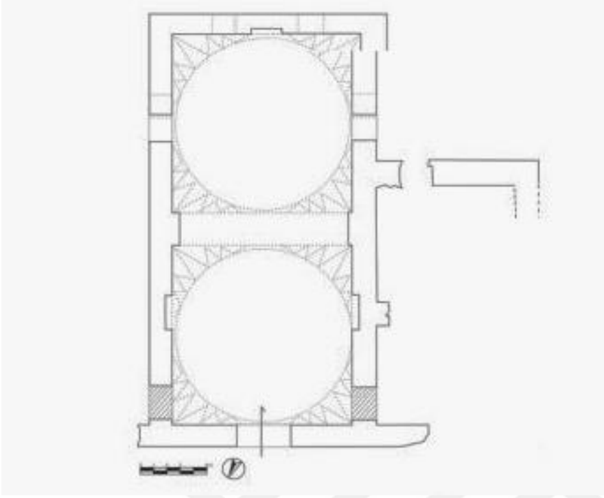
Şekil 12 Bilecik Orhan Gazi İmareti Planı (Türkan Acar)
