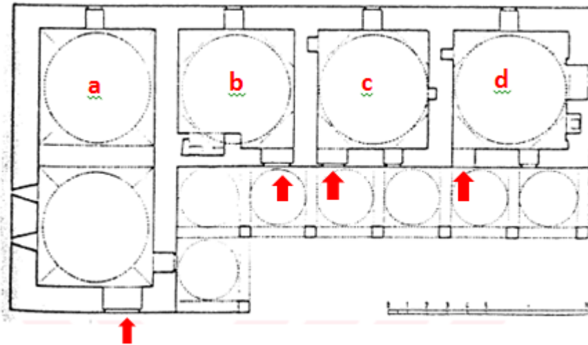
Şekil 64 İmaretin Planı (Birsen Parlar)
