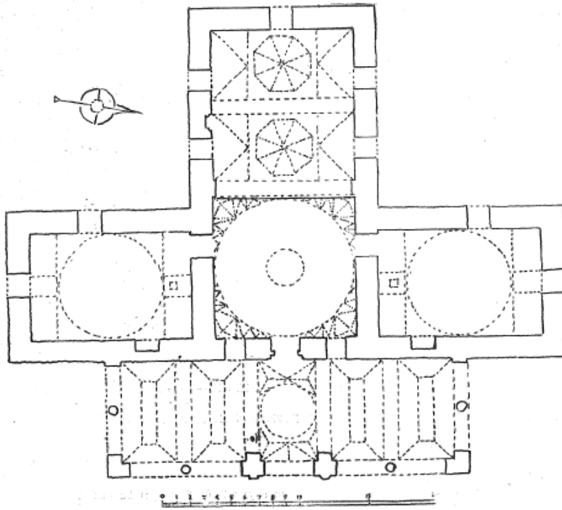
Şekil 11 Nilüfer Hatun İmareti Planı (Semavi Eyice)
