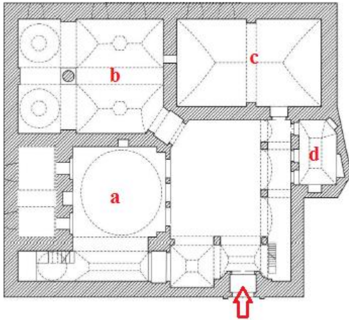
Şekil 145 İmaretin Planı (P. Sürmen'den)
