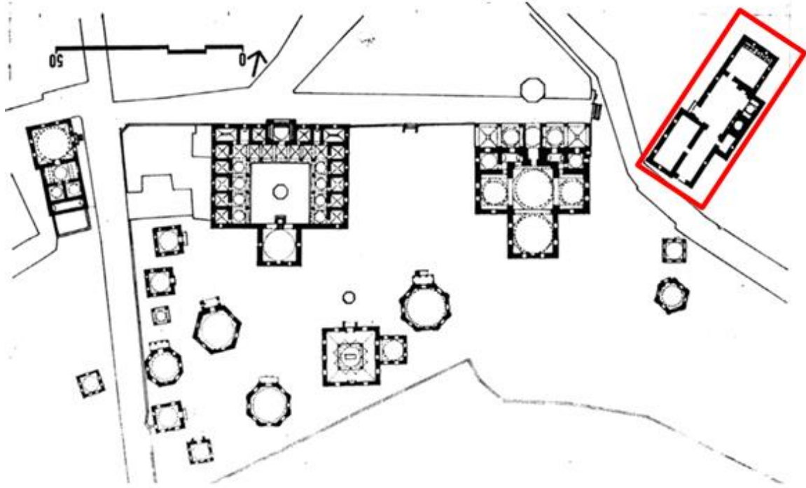
Şekil 16(Muradiye Külliyesi Vaziyet Planı)
